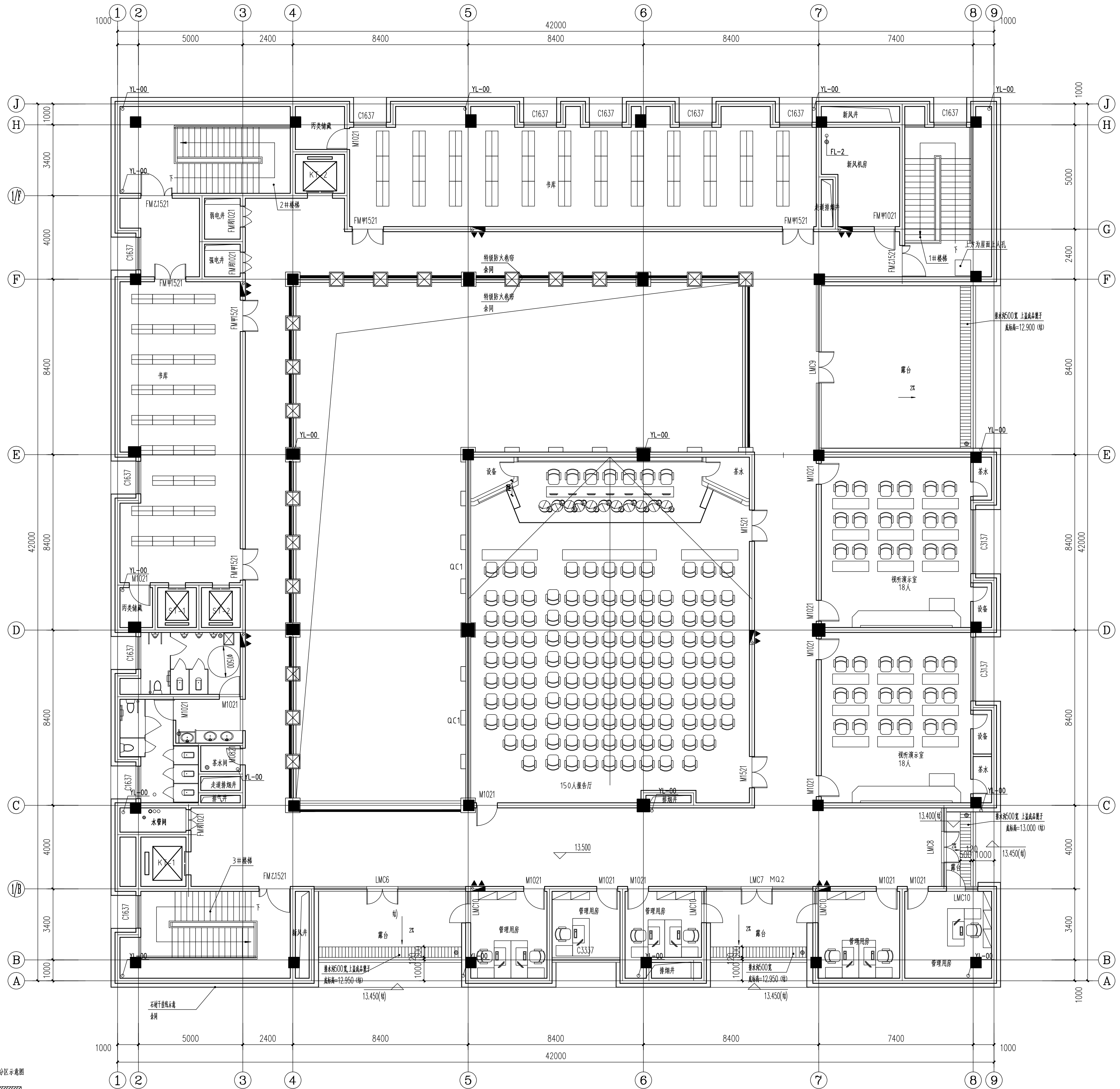
四层平面图 1:100
