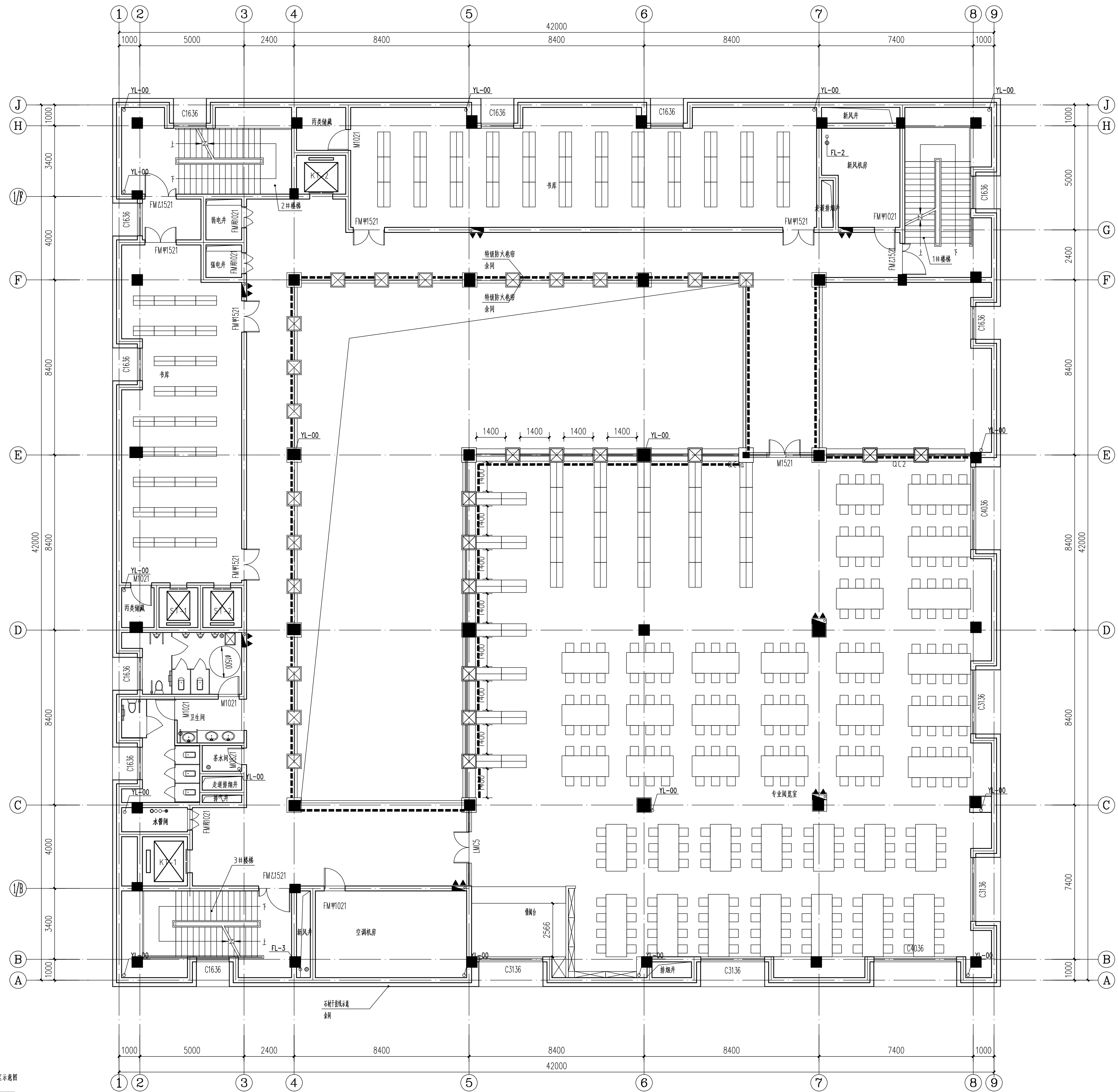
三层平面图 1:100
